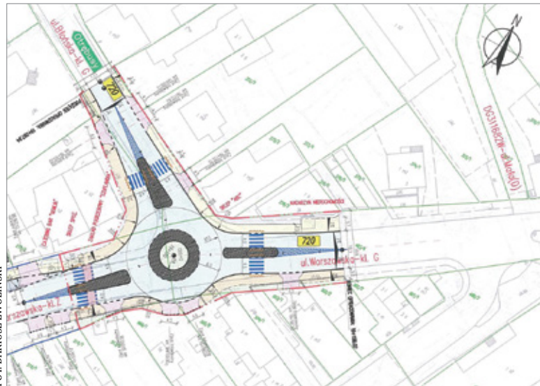
Wstępne opracowanie przebudowy skrzyżowania
